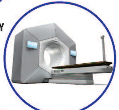
640 SLICE MDCT
